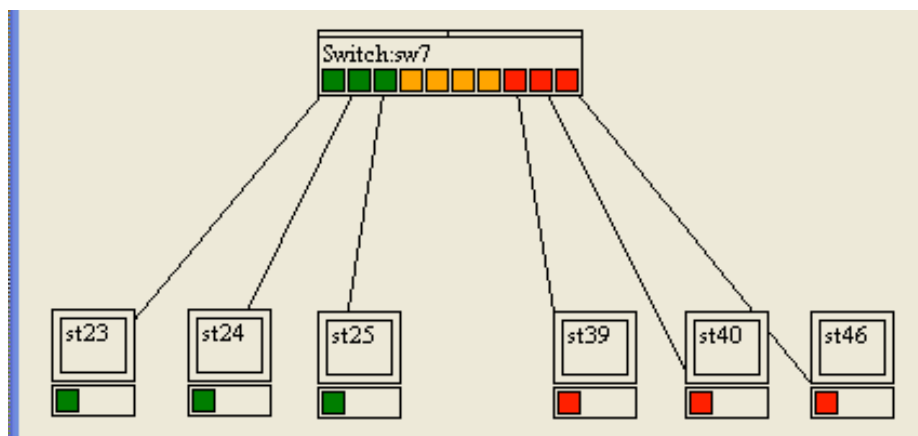
Figure 7: 2 VLAN sur un même switch
